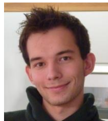
Lorenz
